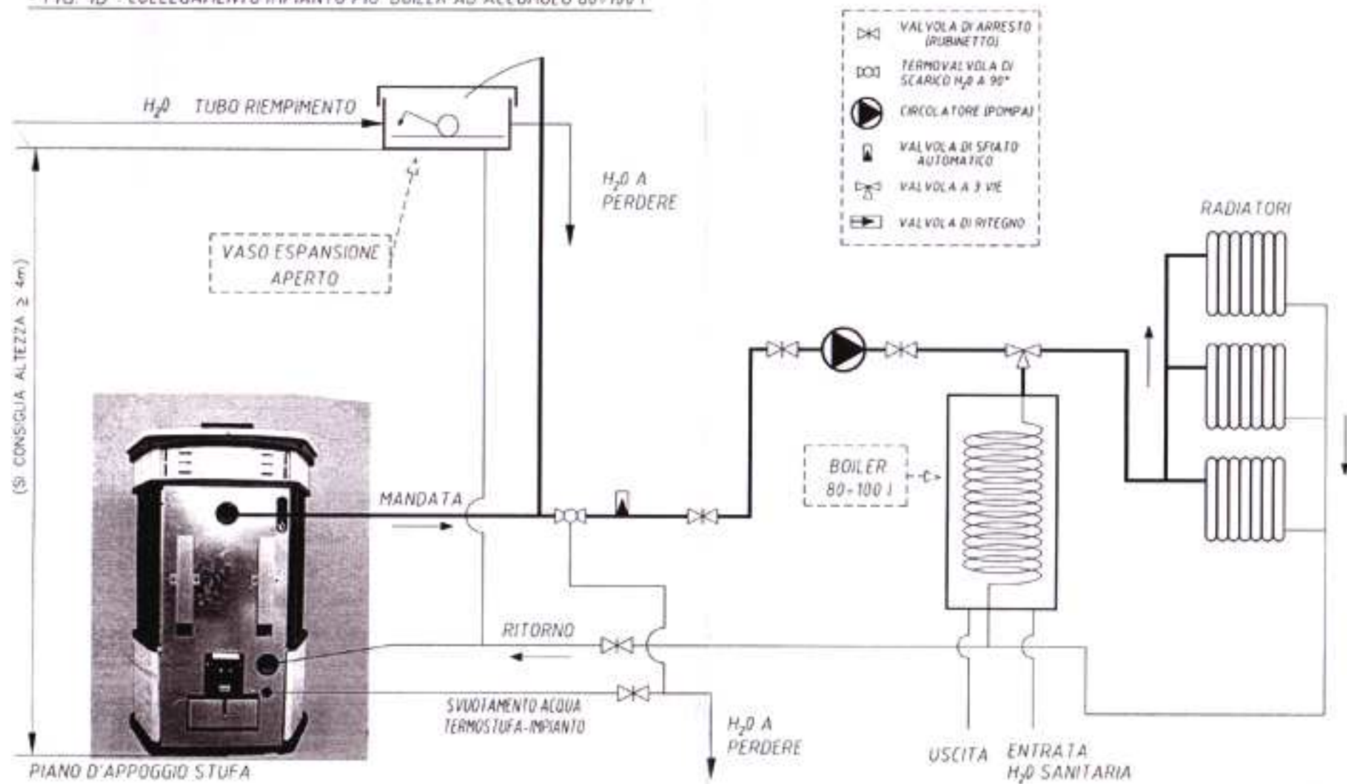
FIG. 1B : COLLEGAMENTO IMPIANTO PIU' BOILER AD ACCUMULO 80-100 l
