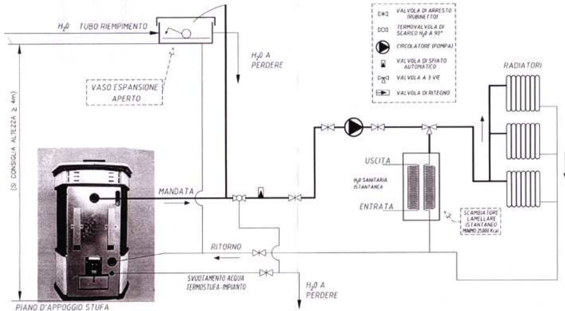
FIG. 1C COLLEGAMENTO IMPIANTO E SCAMBIATORE RAPIDO PER ACQUA CALDA ISTANTANEA
